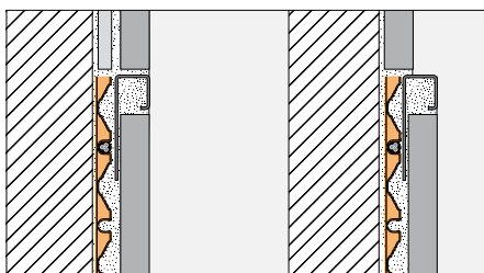
Esempio di posa: zona scaldata contraddistinta visivamente tramite Schlüter®-QUADEC
