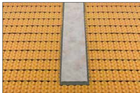
Giunzione impermeabilizzata con Schlüter®-KERDI-KEBA
